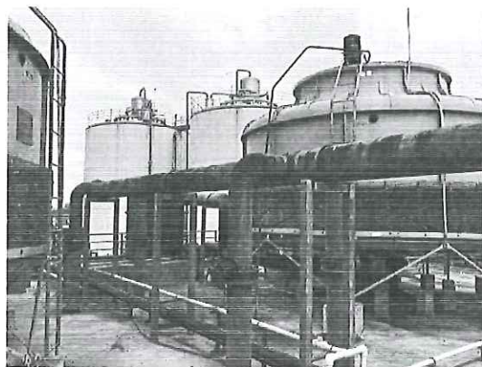
渗滤液处 理站设备 设施锈蚀 情况
