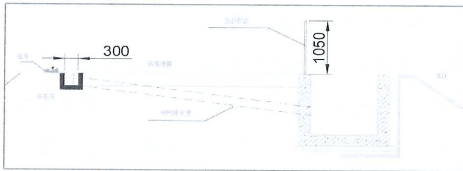
剖面图 1
