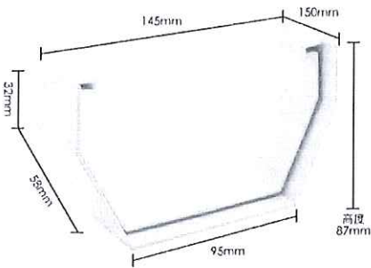
160天沟接头
